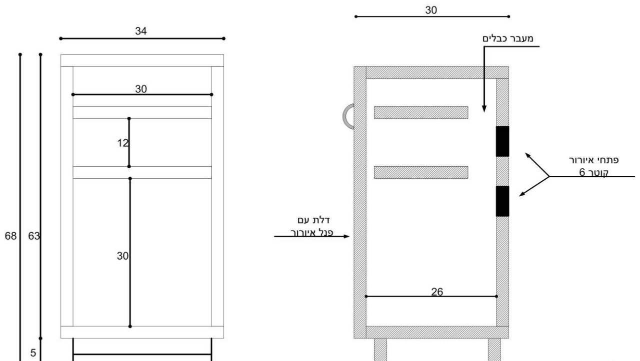
חזית ( ללא הדלת)
