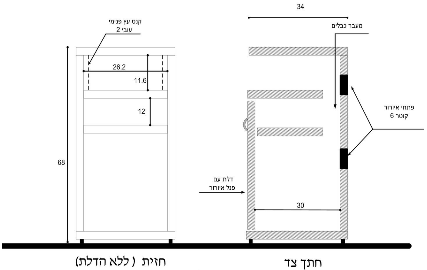
ארון מצבר ספק לחדרים הכוללים קשר
